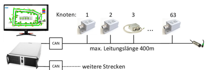
peristop® - IMS 3D-Beschleunigungssensoren
